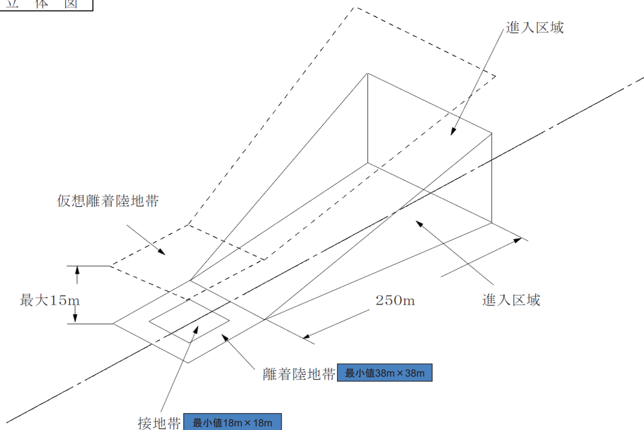
立体図
