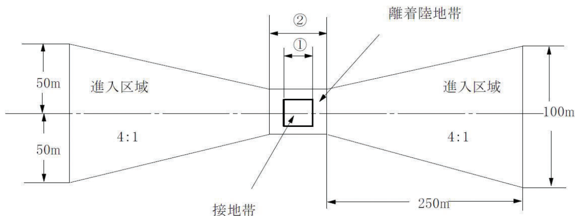
平 面 図
