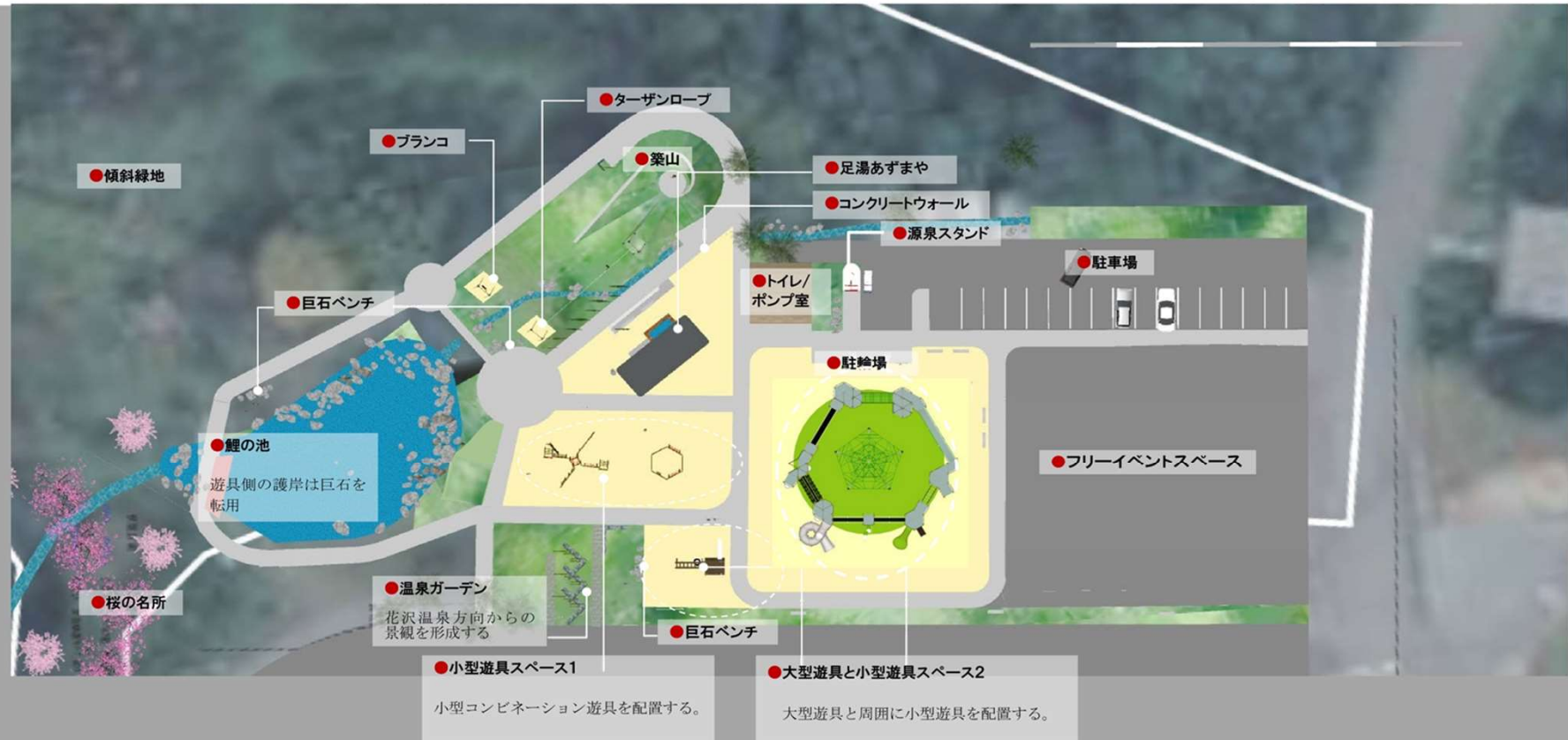
花沢公園再整備 あそびの中心ゾーン計画平面図 S=1:500
