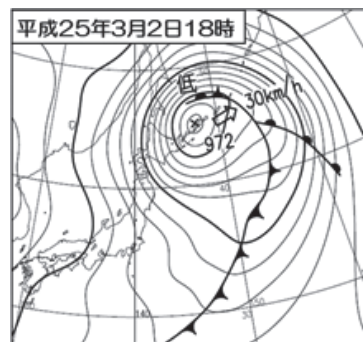
平成25年(2013年)3月2日 18時の地上天気図 (暴風雪により、北海道内で9名の方が亡くなりました)
